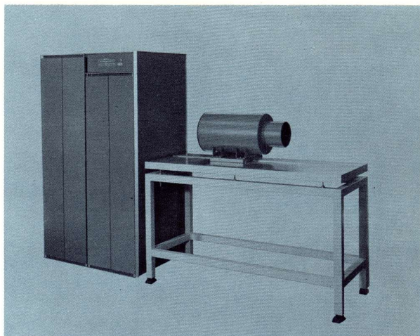
Ultra-Precision CRT Display
